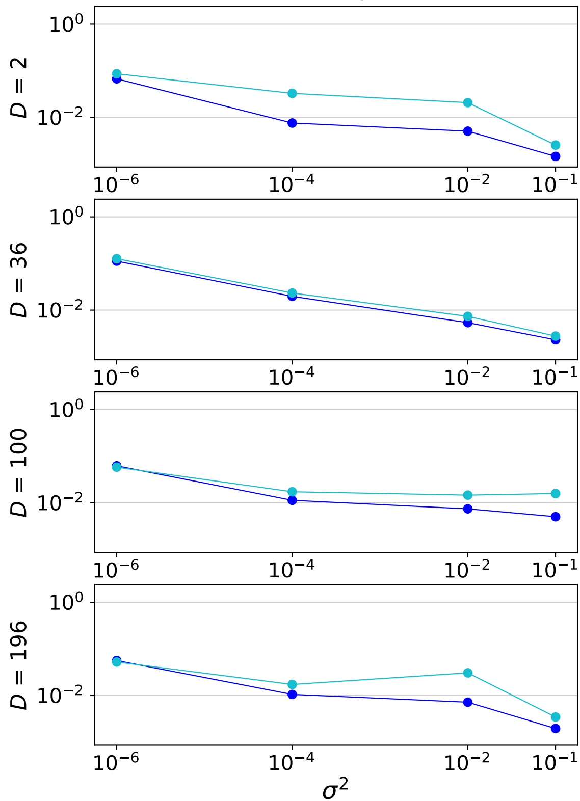
KL Div / D
