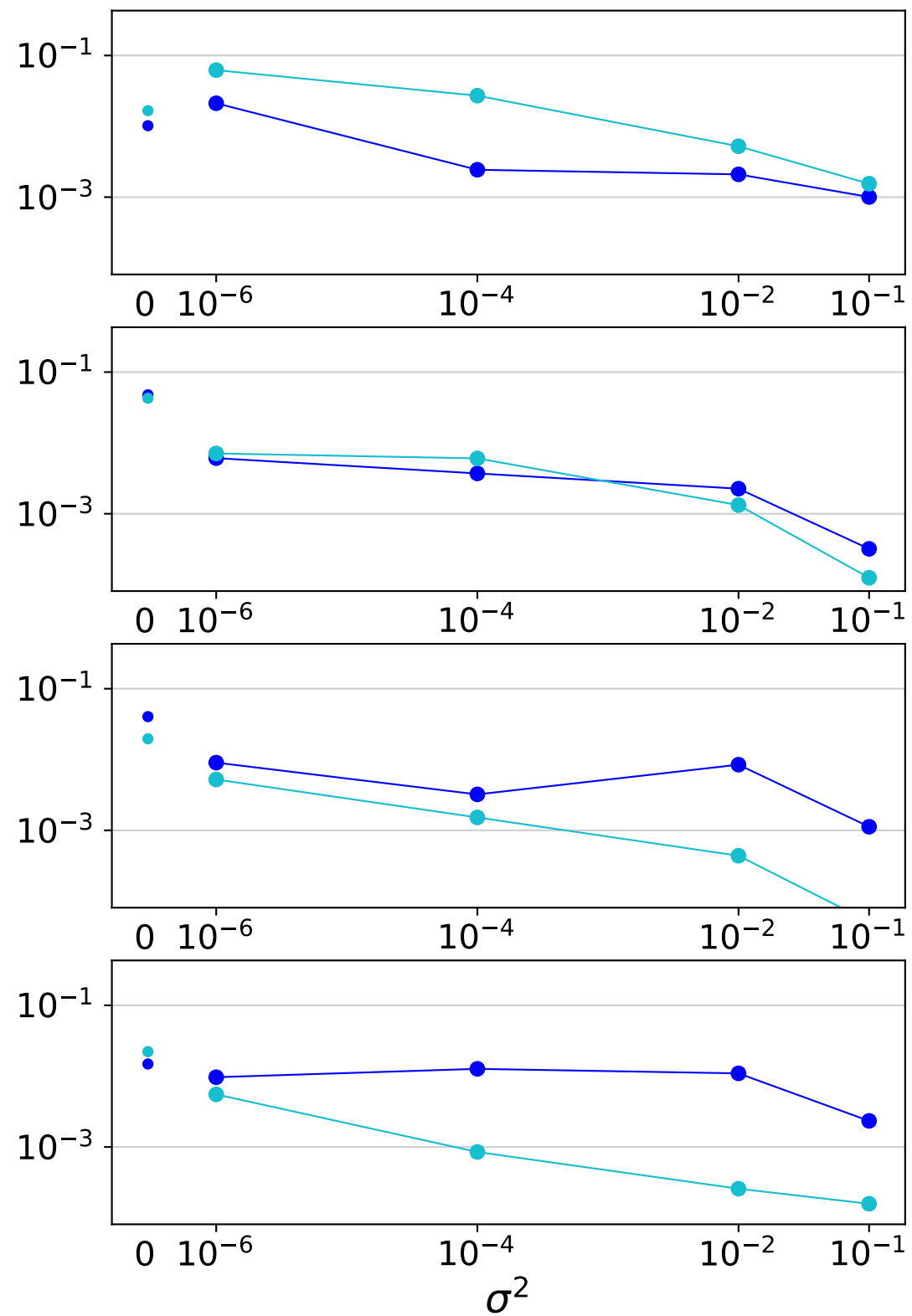
KL Div on Manifold
